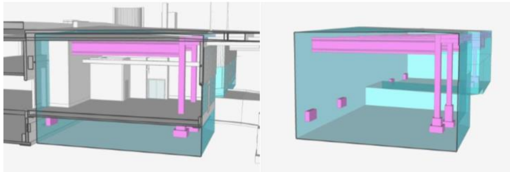
10.5 Tvärsnitt ur modellen för pilotområdet där 3D-fastighetens gränser är markerade i blått och rättigheter i rosa. Bilden t.v. visar fastighetsbildningsmodellen med byggnadsinformation, gränser och rättigheter, t.h. visas registermodellen med endast gränser och rättigheter.
